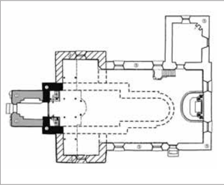
Fig. 5. Landeryds kyrka, Plan förf. och Lars Östlin, efter Tagesson 2006. —Landeryd church
